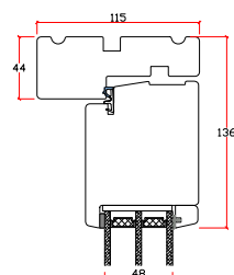
Lodret snit A
