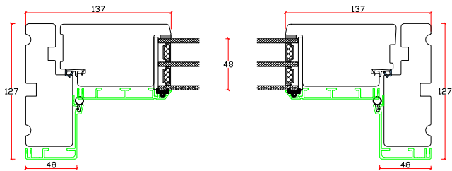
Vandret snit B
