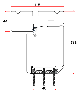
Lodret snit A
