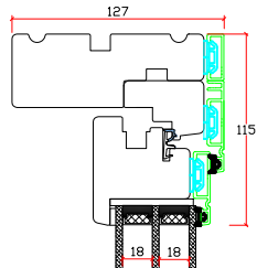
Lodret snit A
