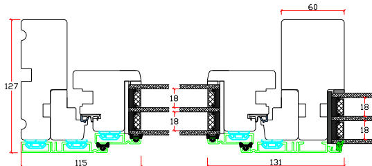
Vandret snit B
