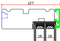
Lodret snit C
