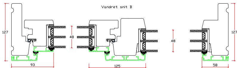
Vandret snit B
