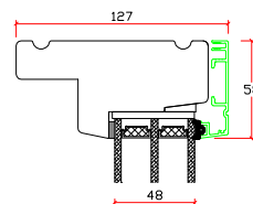
Lodret snit C
