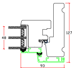
Vandret snit B
