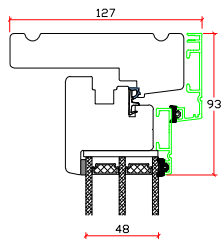
Lodret snit A
