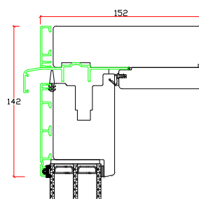
Lodret snit B
