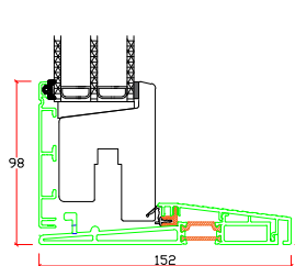
Lodret snit B
