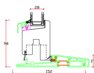
Lodret snit B
