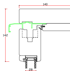
Lodret snit B
