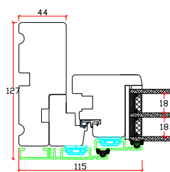
Vandret snit C
