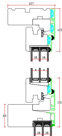
Lodret snit A
