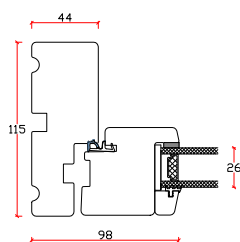
Vandret snit B
