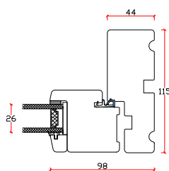
Vandret snit B
