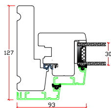
Vandret snit C
