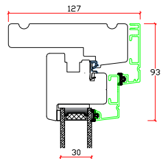
Lodret snit A
