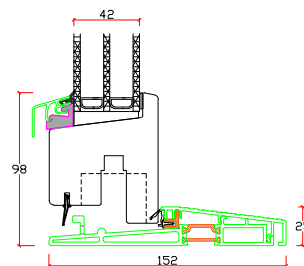
Lodret snit B
