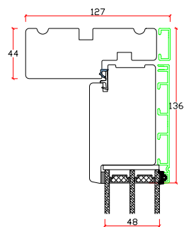
Lodret snit A
